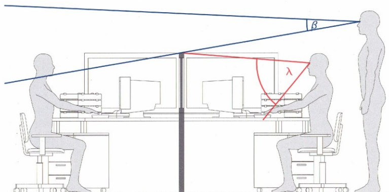
Rys. nr 6. Schemat idealowy wykorzystania ekranów izolacyjnych w pomieszczeniu pracy ogólnej.
