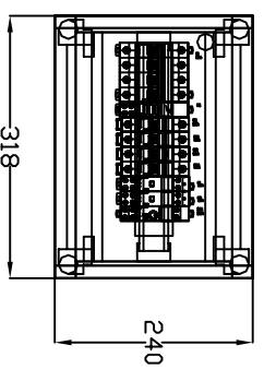
R oświetl. Rozdzielnica na tylnikowa (nedbox)
