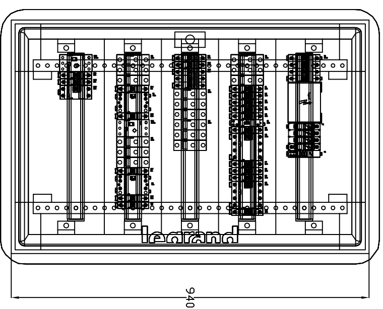
Rozdzielnica RG (typ XL3-160 p/t)
