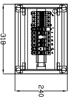
R 1. Rozdzielnica na tylnikowa (nedbox)
