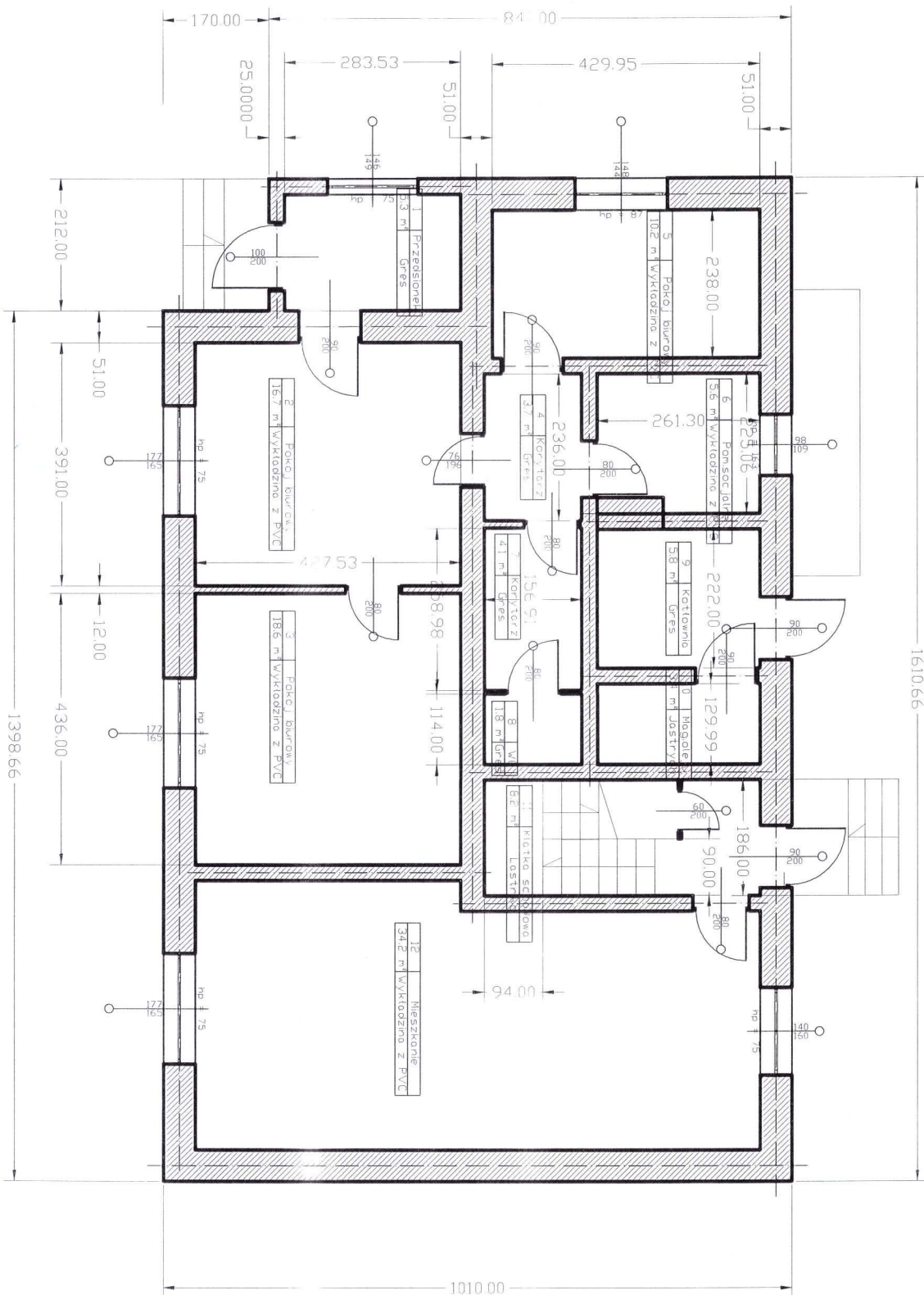
RZUT PARTERU 1:100 - stan istniejący
